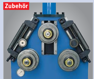
Zubehör ▶ Option Spezial-Richtrollen seitlich, für Winkeleisen
